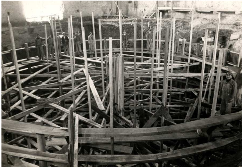
Der 16 m tiefe Guß für die Struktur des zweiten auf Huemul vorgesehenen Reaktors
